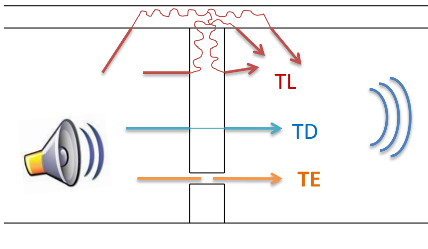
Imagen 1. Vías de transmisión de los ruidos
